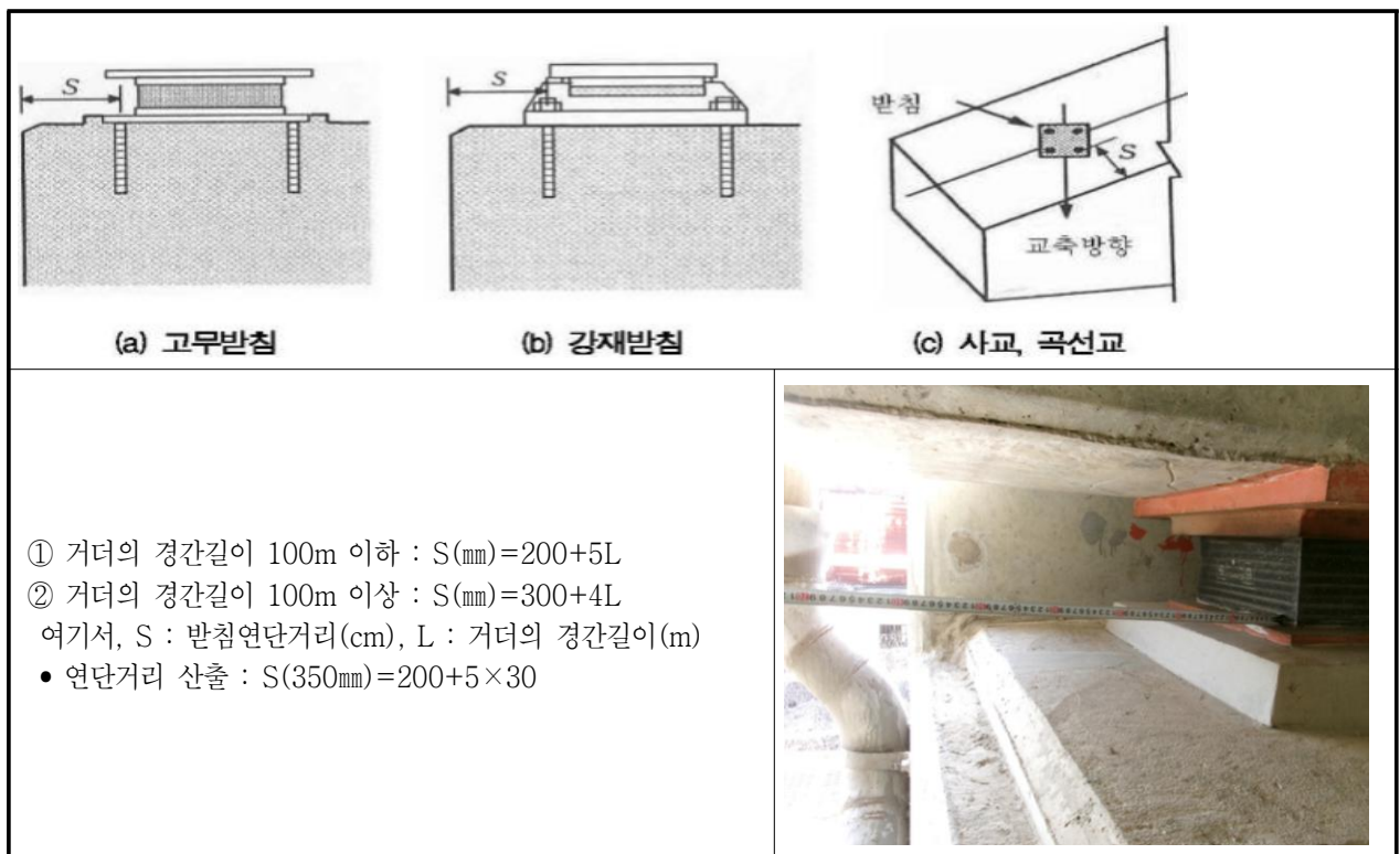
【그림 2.3.2】 도로교설계기준 연단거리 산출방법
