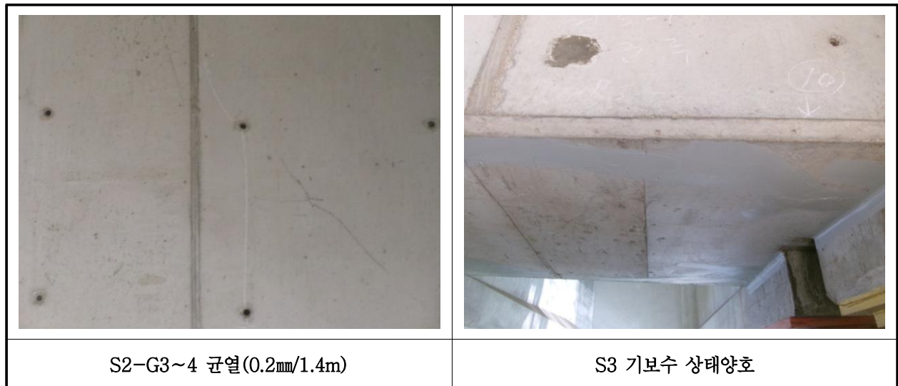
【사진 2.3.7】 가로보 손상현황
