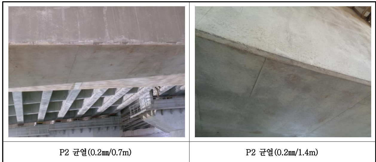
【사진 2.3.11】 교각 손상현황
