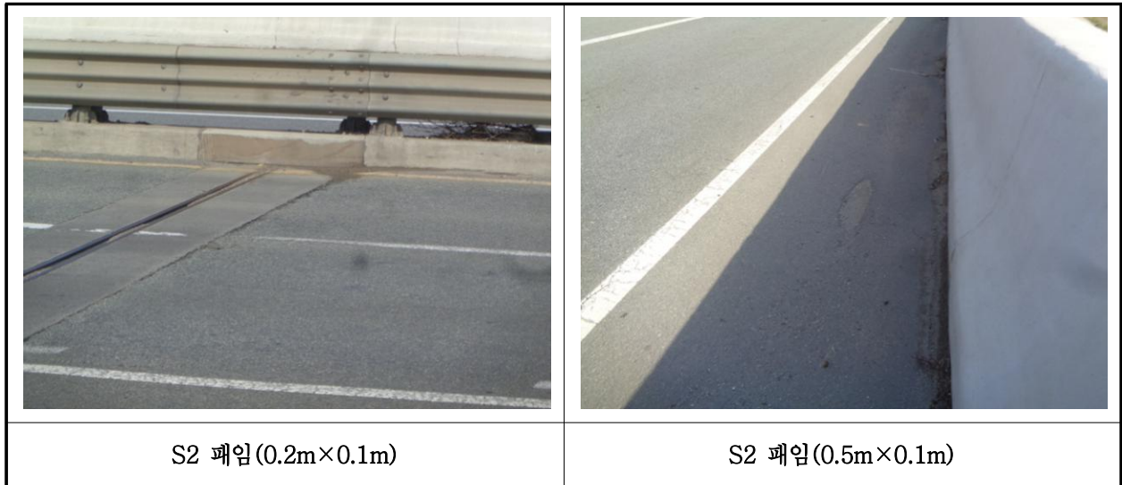
【사진 2.3.18】 교면포장 손상현황
